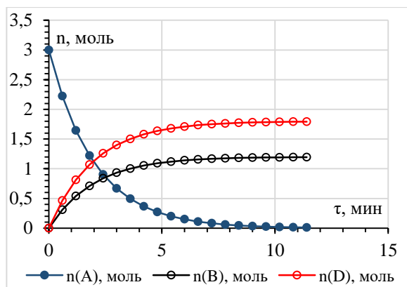
Рисунок 1 – Кинетические кривые для параллельных реакций
